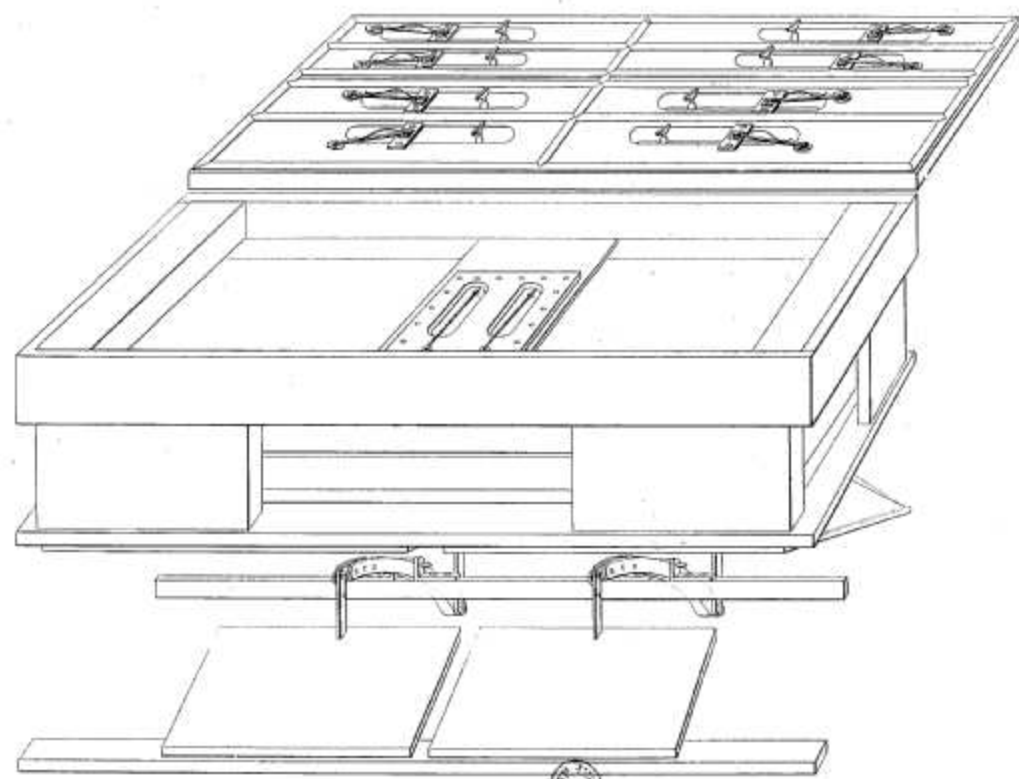
Somme d'un Mélodium sans le système de M. Martin de Sorens.
